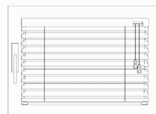
Ausführung mittels Sockel im Glasfalz
