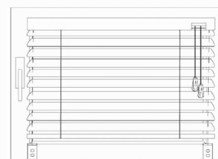
Ausführung mittels Winkel auf den Rahmen
